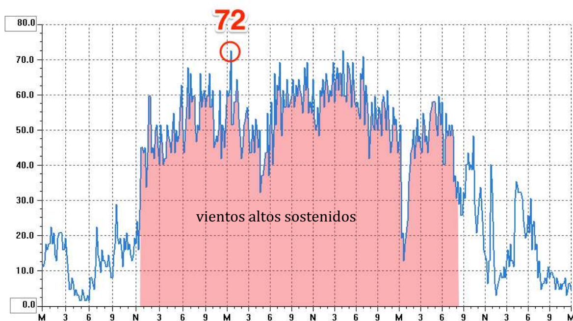
Ráfagas de viento registradas por la estación municipal de SEDAVÍ entre el 19 y el 21/01/20 (en km/h)
