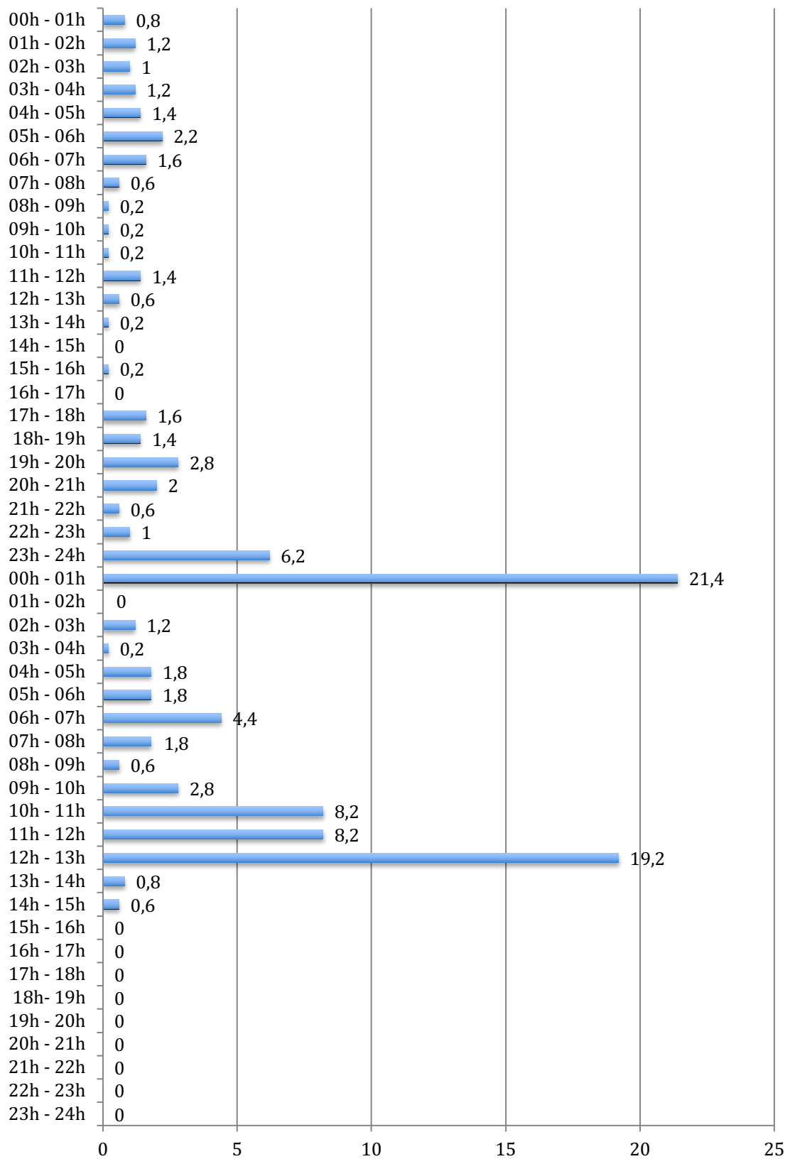
Cantidades de lluvia registradas por horas en SEDAVÍ los días 20 y 21/01/20 (en l/m 2 )
